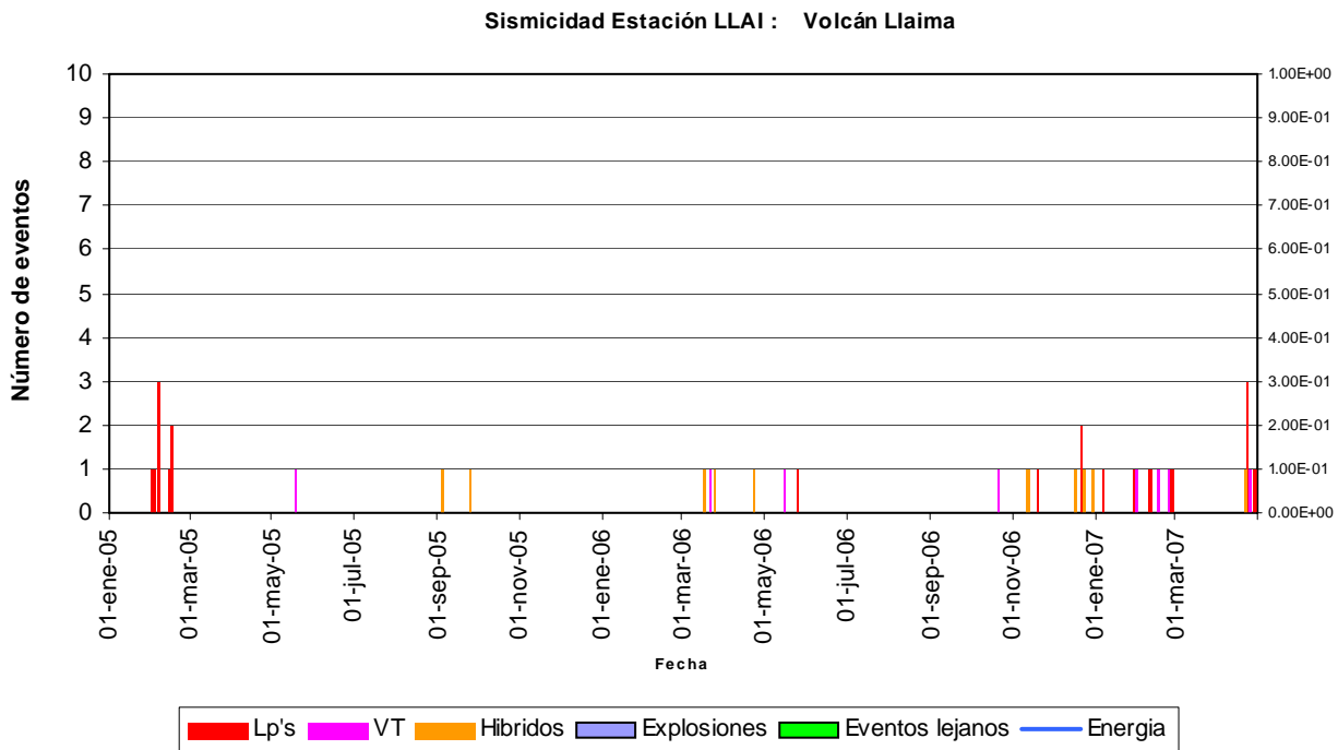
Figura 1. Sismicidad del volcán Llama, período enero 2005 a abril de 2007, registrada por la estación LLAI.
